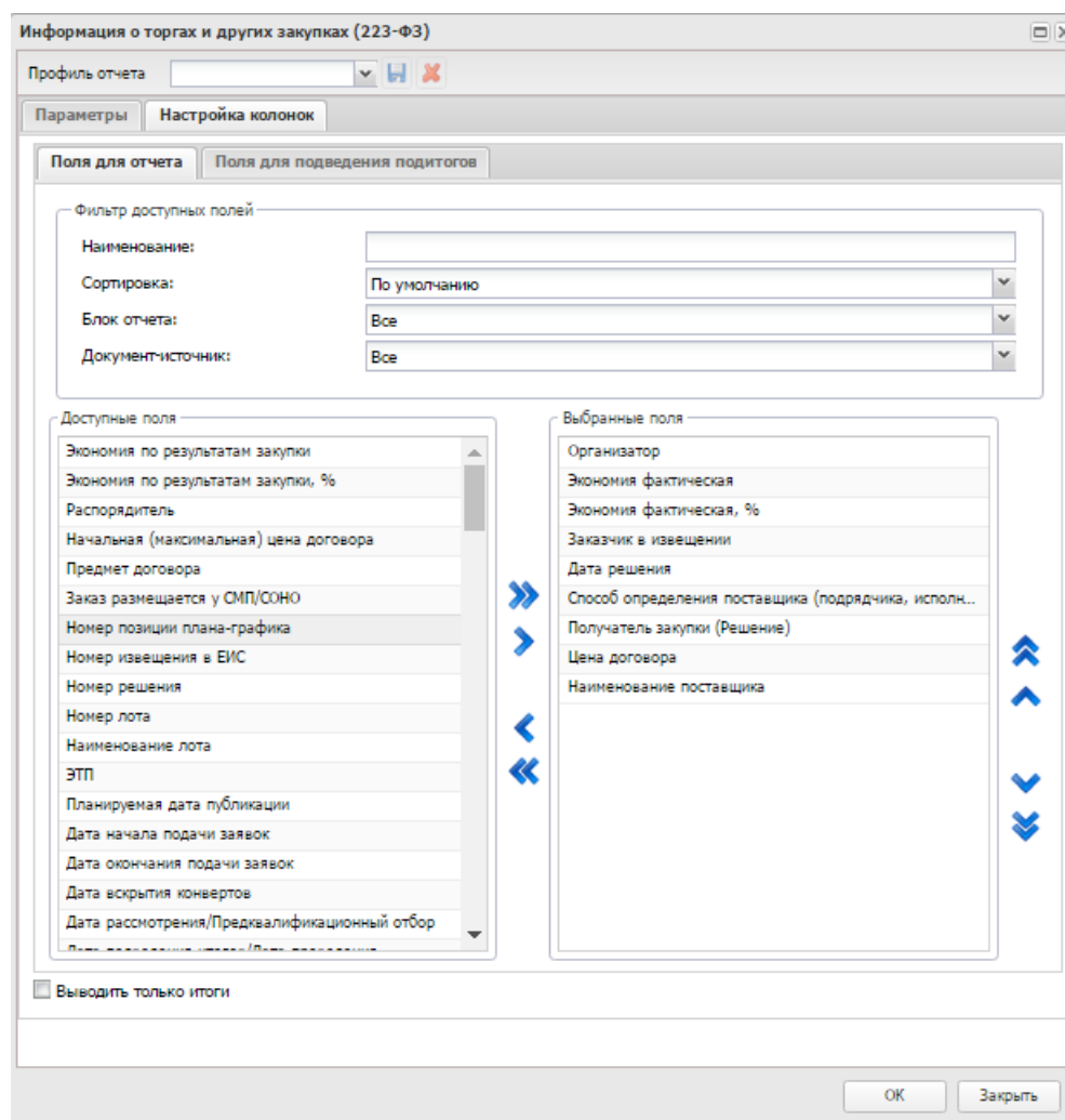
Рисунок 10 – Форма настроек отчета «Информация о торгах и других закупках», закладка «Поля для отчета»
