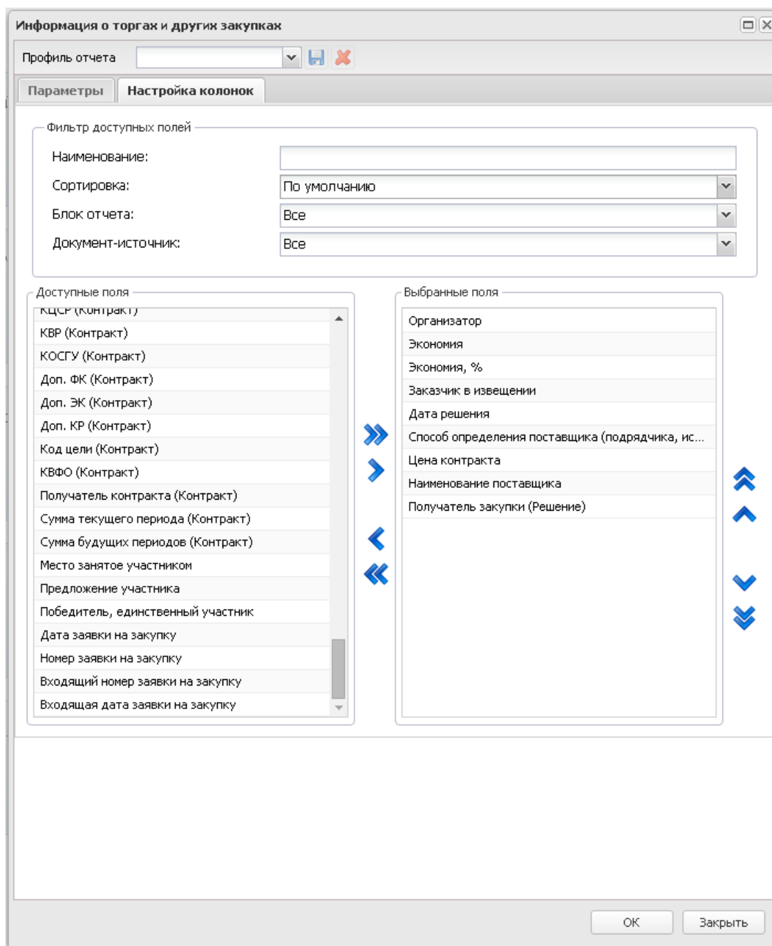
Рисунок 7 – Форма настроек отчета «Информация о торгах и других закупках», закладка «Настройка колонок»
