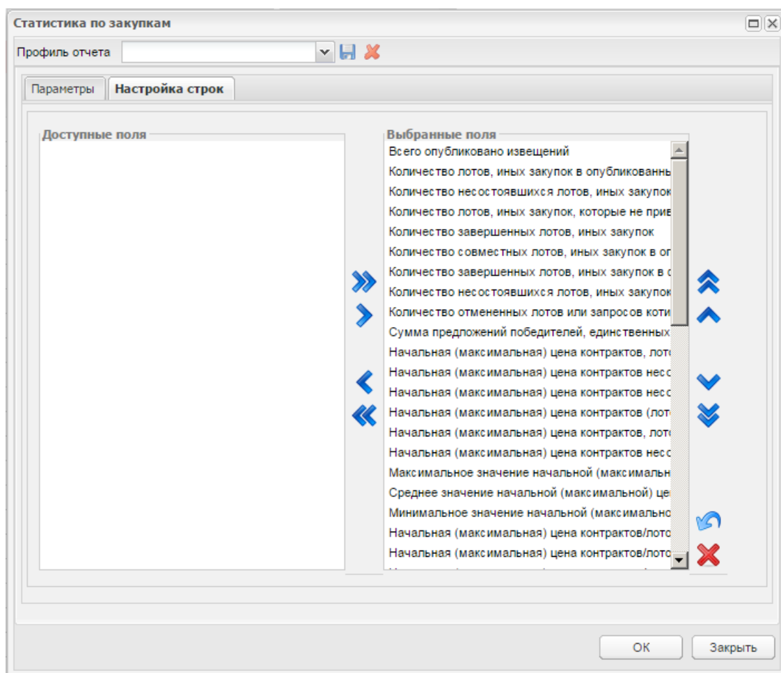
Рисунок 13 – Форма настроек отчета «Статистика по закупкам», закладка «Настройка строк»
